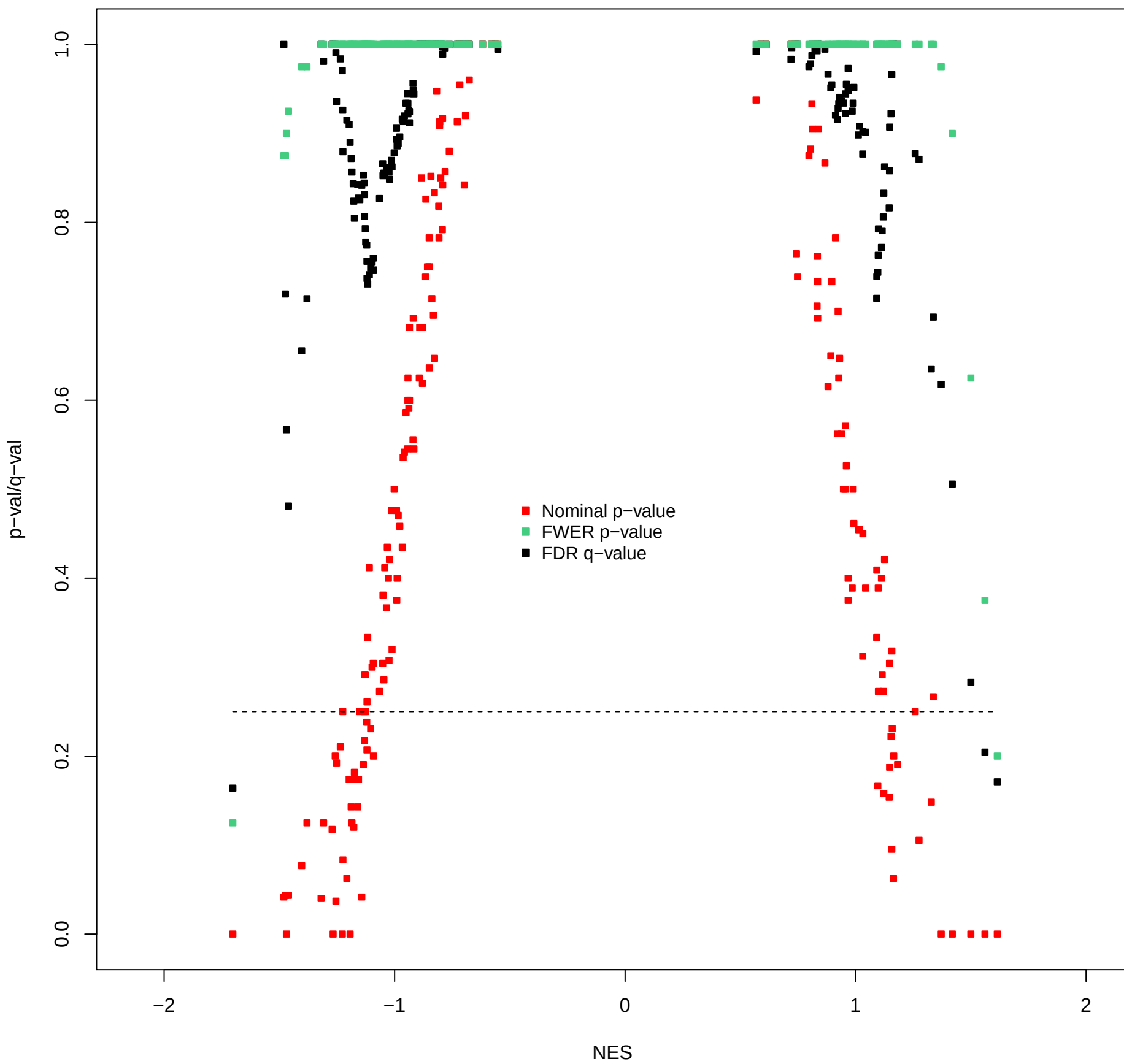
p-values vs. NES
